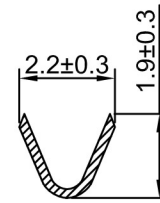
A-A SECTION
